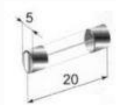
Pojistka trubičková
